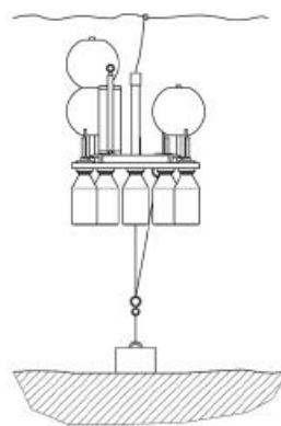
Multi Limnos 安装示意图
